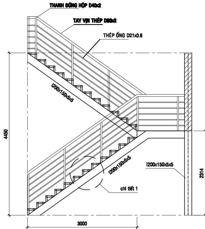
MẶT ĐỨNG CẦU THANG
