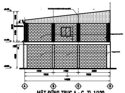
MẶT ĐỨNG TRỰC A - C TL 1/100
