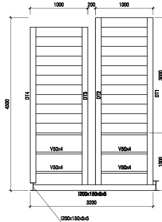
MẶT BẰNG KẾT CẤU CẦU THANG SL:01
