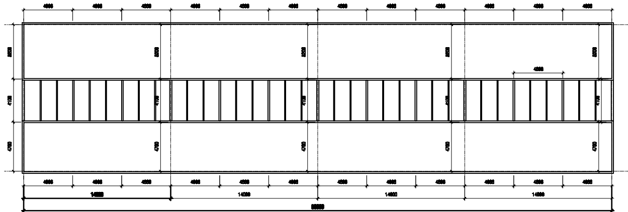
MẶT BẰNG TRẦN TẦNG TRỆT HIỆN TRẠNG
