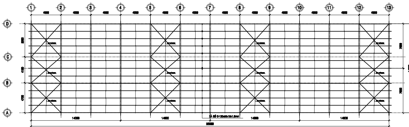
MẶT BẰNG XÀ GỖ MÁI - GIẰNG MÁI
