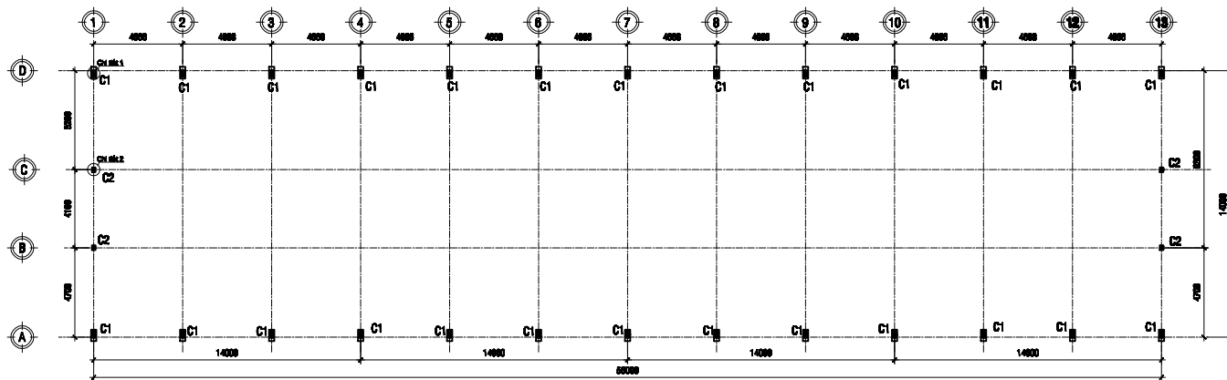
MẶT BẰNG ĐỊNH VỊ CỘT LẦU 1
