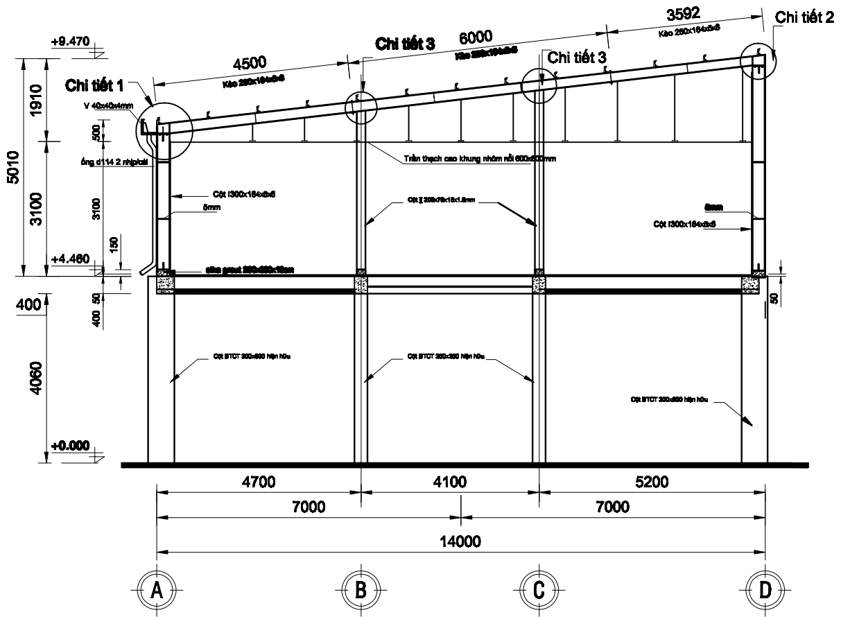
KHUNG KÈO K1 TL 1/100
