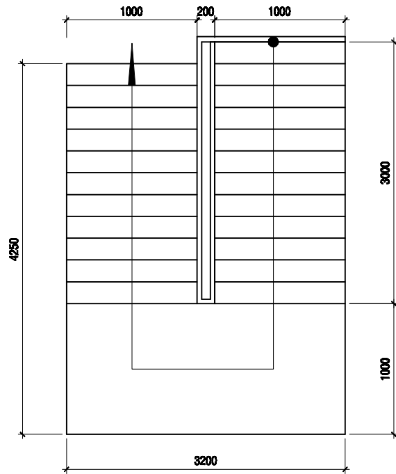
MẶT BẰNG CẦU THANG SL:01
