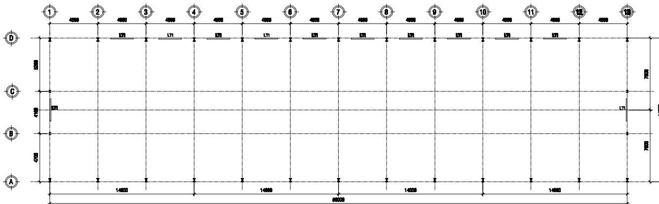
MẶT BẰNG LANH TÔ LẦU 1
