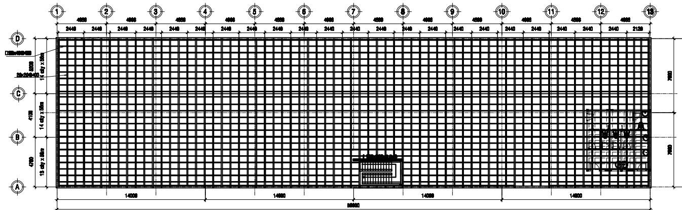
MẶT BẰNG BỐ TRÍ HỆ KHUNG ĐỖ TẤM CEMBOARD 18mm LẦU 1
