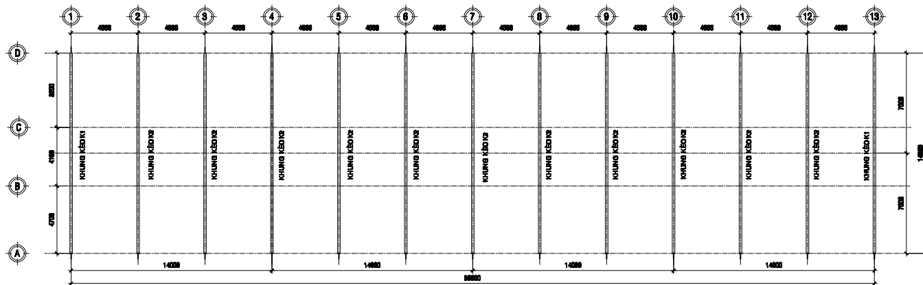
MẶT BẰNG BỐ TRÍ KHUNG KÈO MÁI
